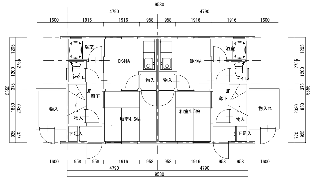
現況 1階平面図
