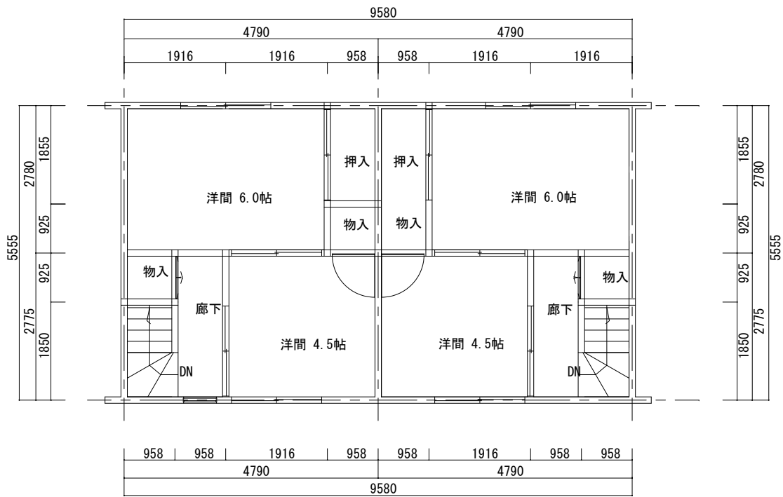
改修後 2階平面図
